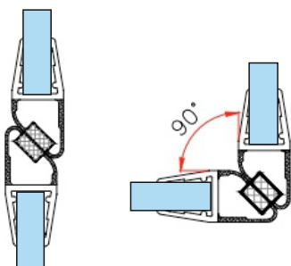
магнит 90/180 гр.
