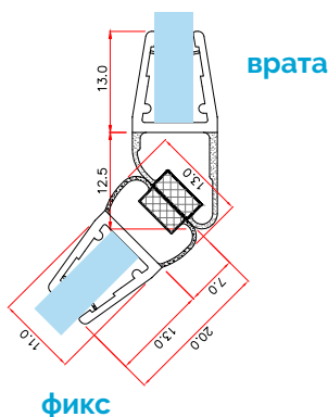
магнит 135 гр
